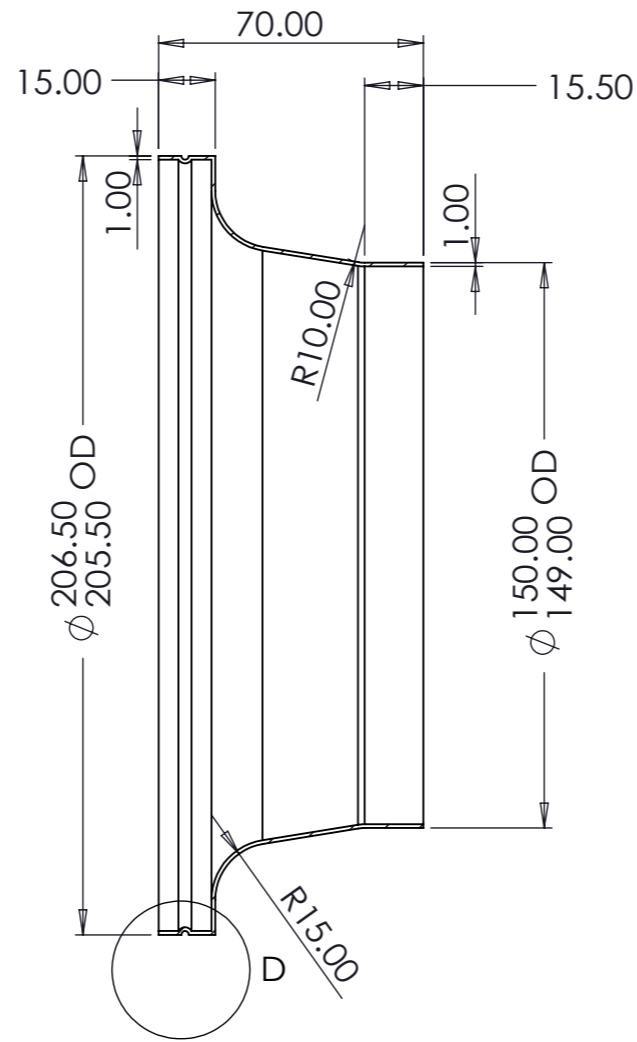
SECTION A-A SCALE 1 : 2
